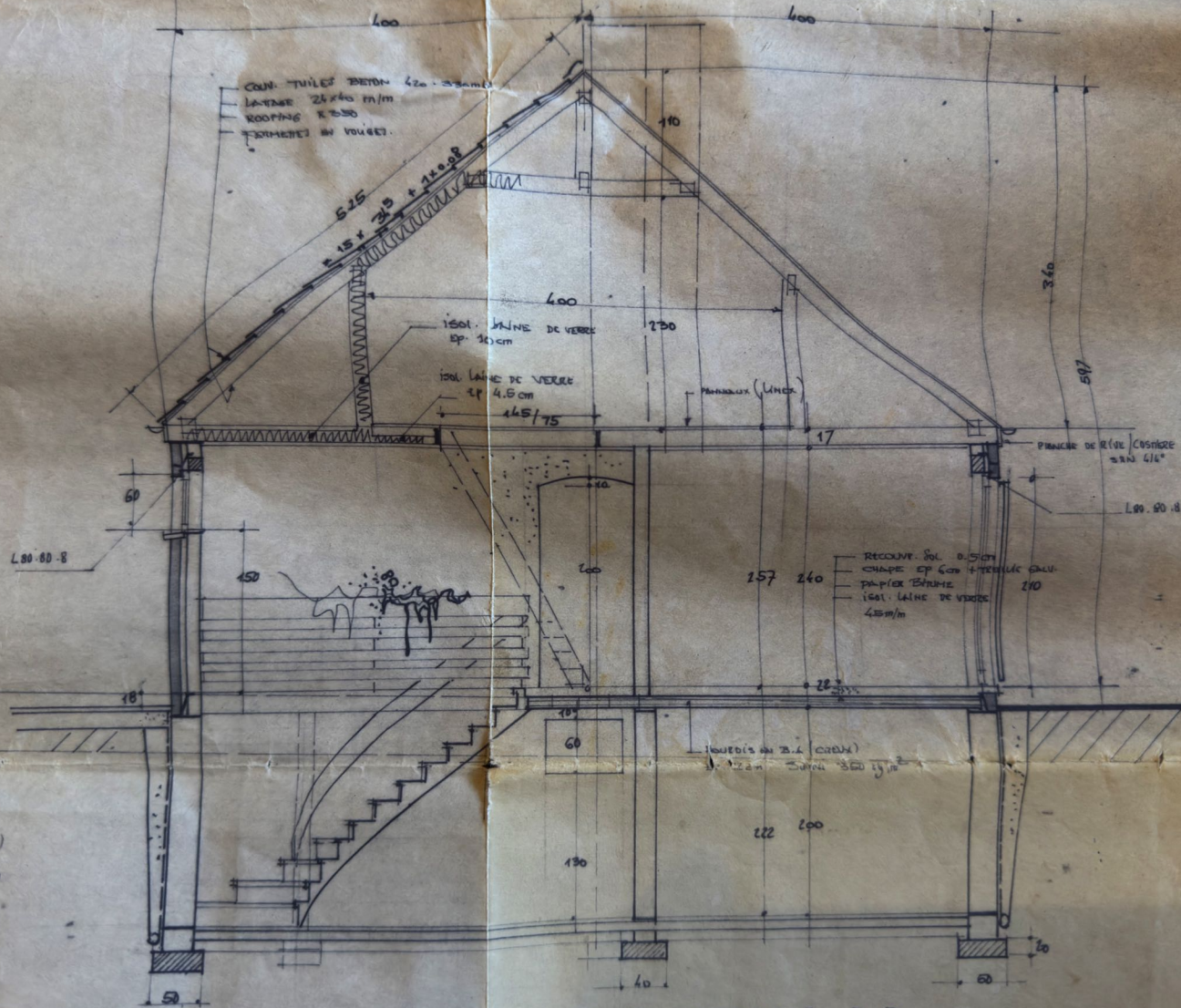
-COUPE TRANSVERSALE: B-B
